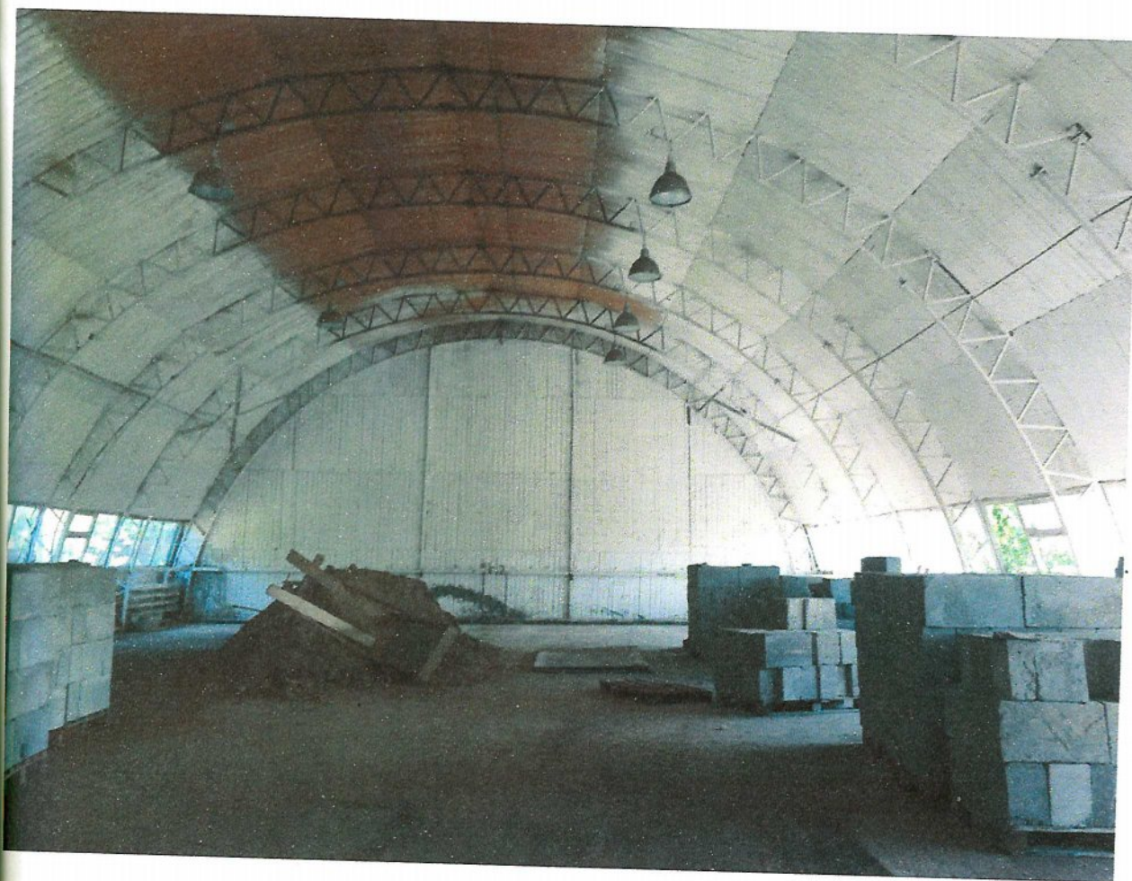
Фото 6. Одноэтажный металлический склад
